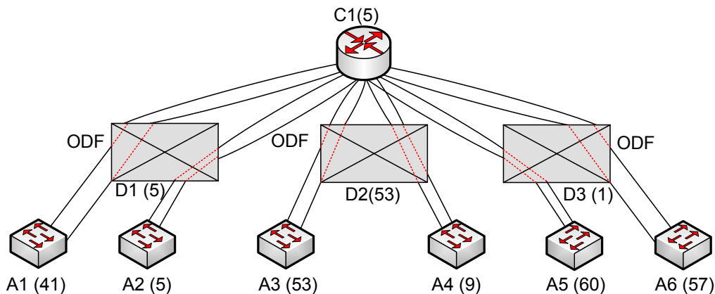
Σχήμα 1: Λογική αναπαράσταση Δικτύου Διανομής του MAN Κέρκυρας
